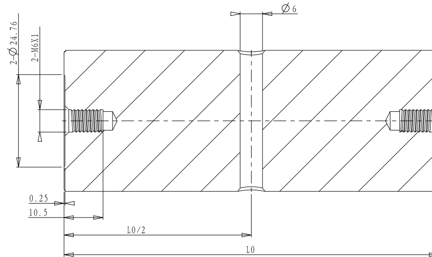
截面 A-A
